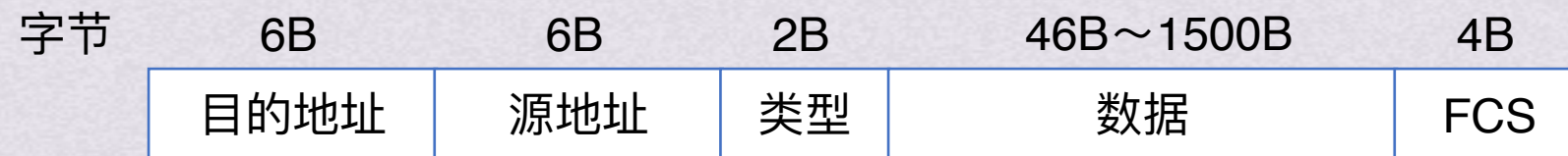
以太网V2标准MAC帧格式
